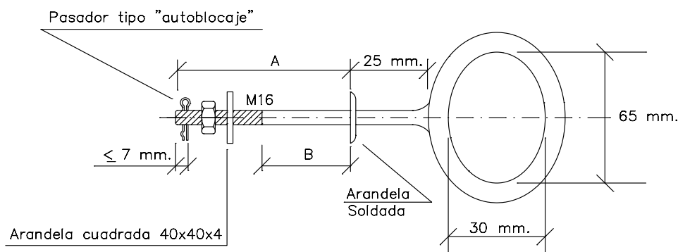
TORNILLO PASANTE DE ANILLA OVALADA PARA LINEA DE VIDA (Figura 6)
