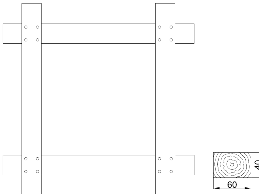
Figura 2 Cuna para el transporte de bobinas
